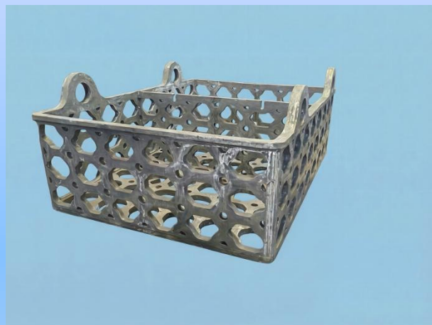
料 筐
